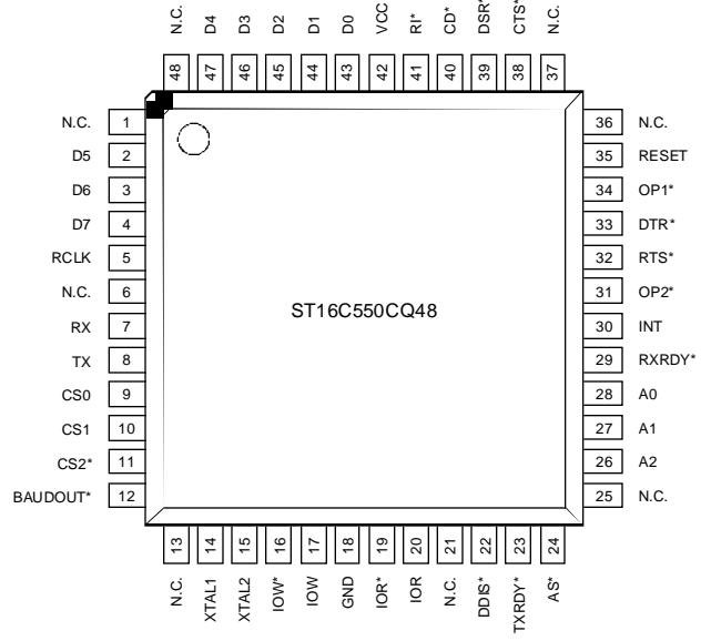
48 Pin TQFP Package
